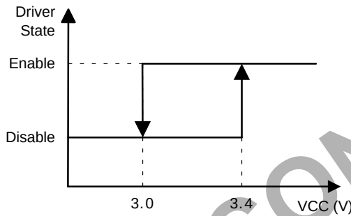
Figure 27. UVLO
