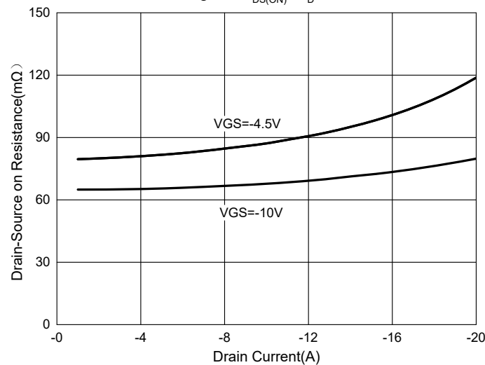
Fig. 4 - R_{DS(ON)} - I_D
