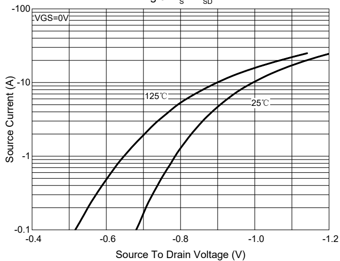
Fig.9 - I_S - V_{SD}
