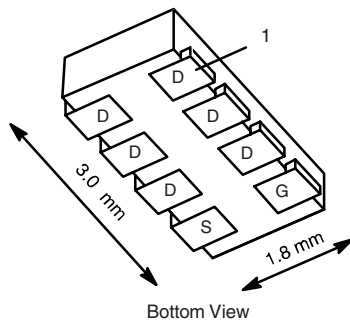
1206-8 ChipFET®
