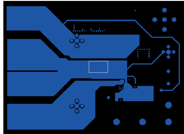
Fig. 12 - Inner Layer2
